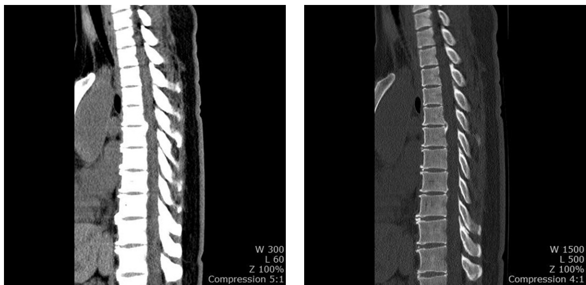
Fig. 3. T-spine CT(2014.9.10).
